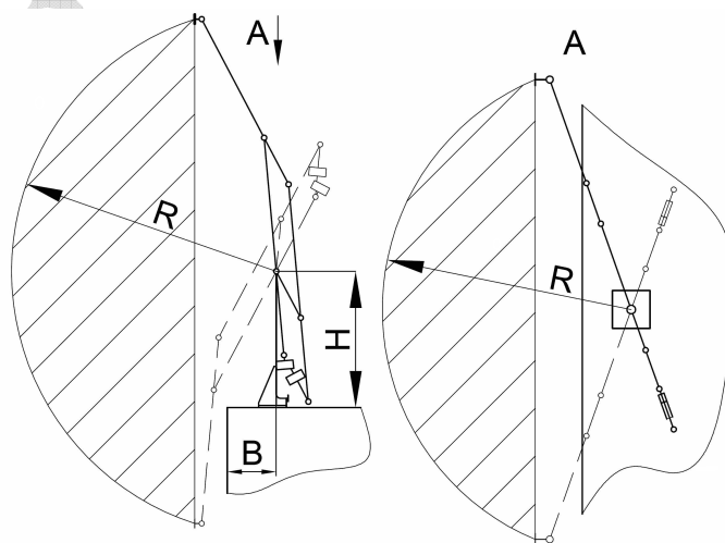
Рисунок 1 – Расположение стендера на причале.
