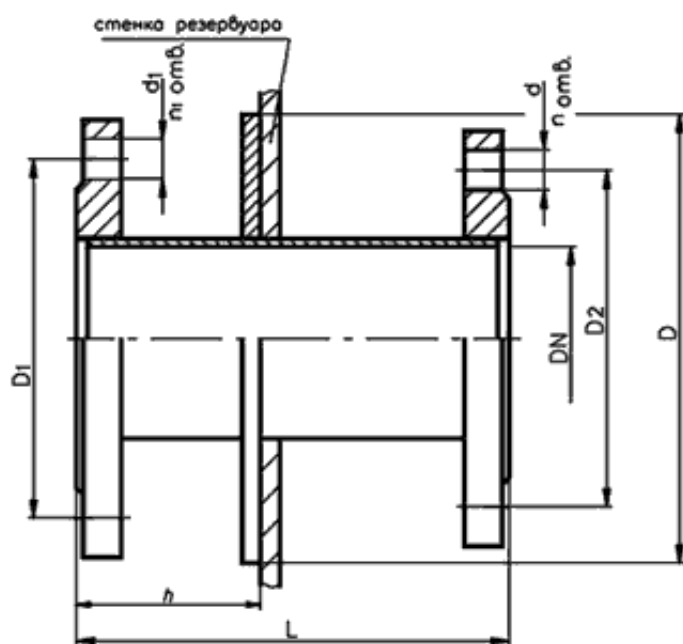
Общий вид приёмо-раздаточного патрубка (ППР-80...ППР-350)
