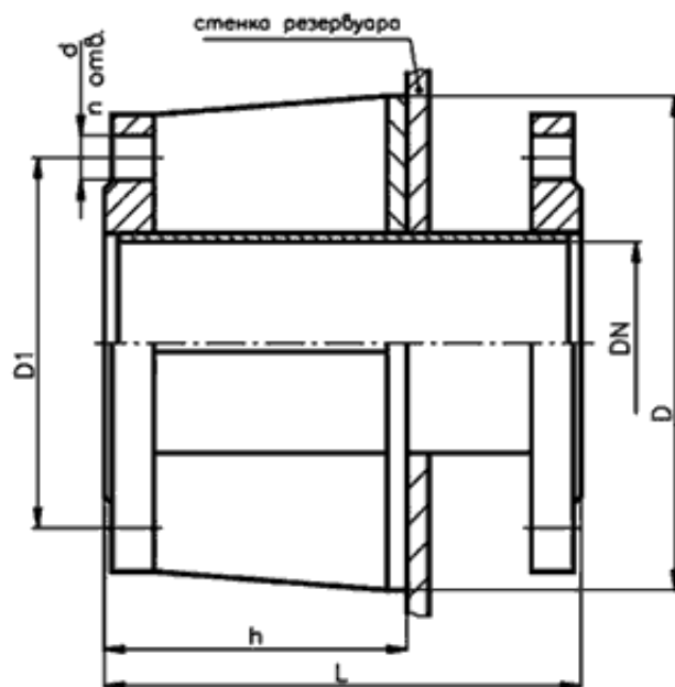
Общий вид приёмо-раздаточного патрубка (ППР-400...ППР-600)
