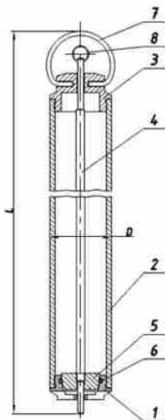
Пробоотборник ПОМ-1
