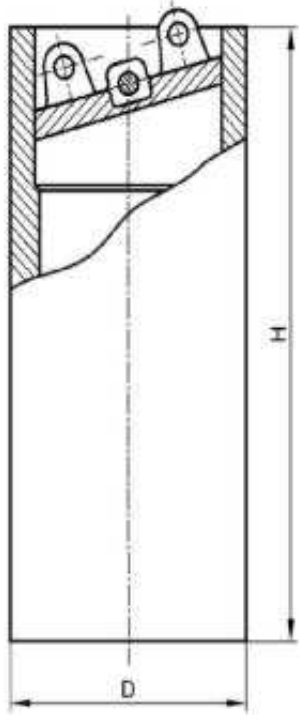
Общий вид пробоотборника ПО-1
