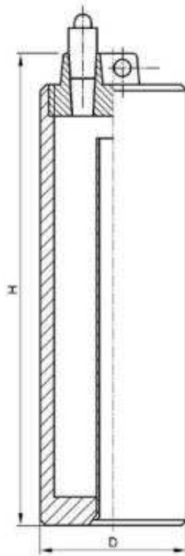
Общий вид пробоотборника ПО-2
