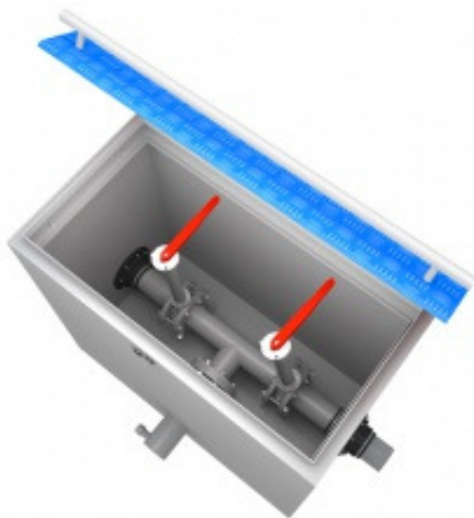
Тех. отсек переключения аварийных проливов с кранами шаровыми Ду 100
